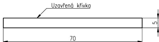
Obrázek 3.28: Uzavřená křivka
