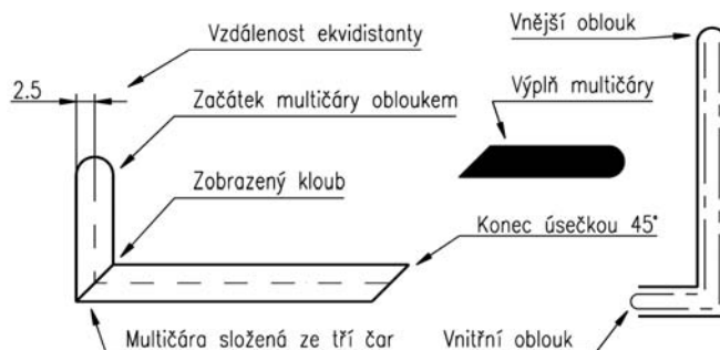
Obrázek 3.40: Parametry multičáry
