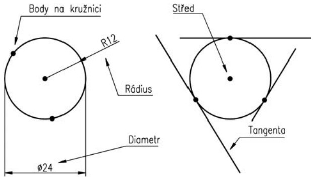
Obrázek 3.6: Parametry kružnice
