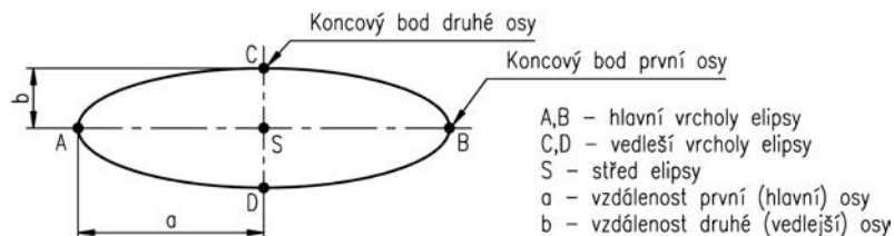
Obrázek 3.17: Parametry elipsy
