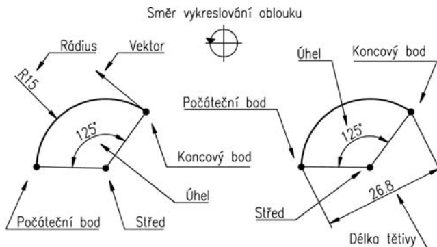
Obrázek 3.14: Parametry oblouku
