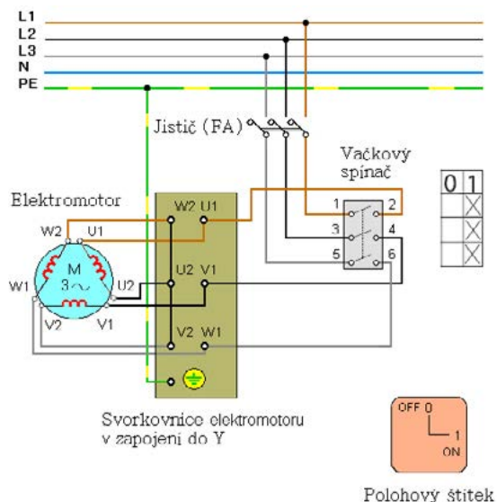
Obrázek 1.1 Schéma zapojení
