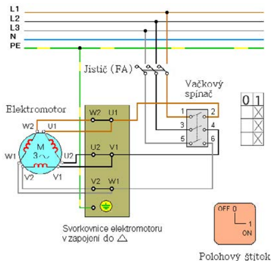
Obrázek 1.2 Schéma zapojení
