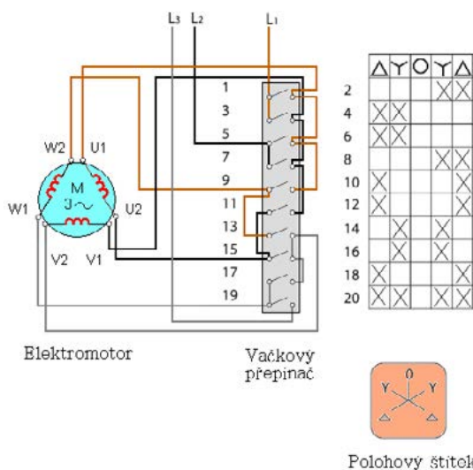
Obrázek 1.8 Schéma zapojení
