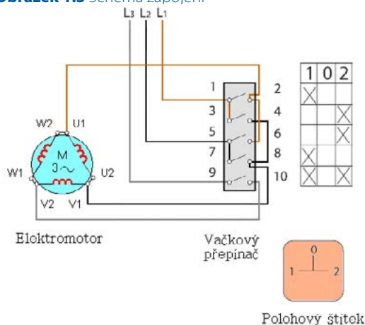
Obrázek 1.3 Schéma zapojení
