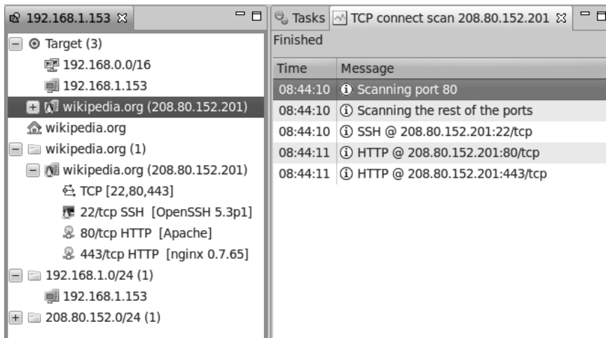
Obrázek 2.5 Netifera GUI
