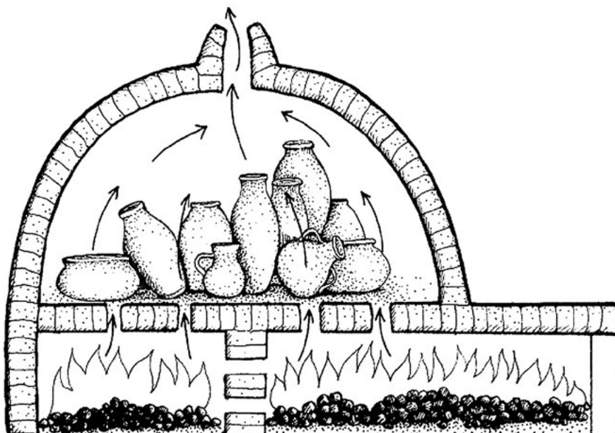
Hrnčířská pec v Anglii (podle Allen 2009)
