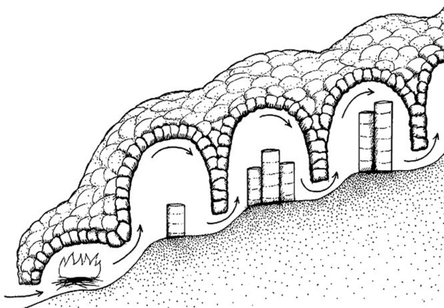
Hrnčířská pec v Číně (podle Allen 2009)
