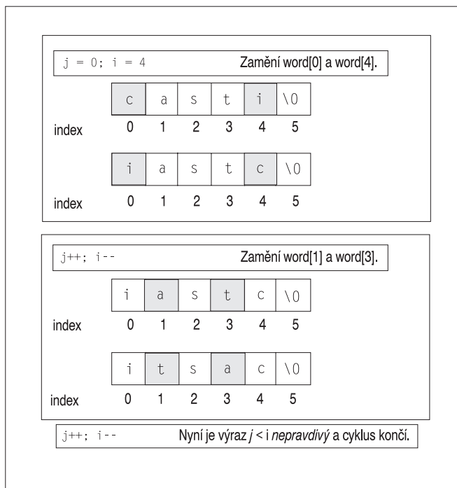
Obrázek 5.2 Obrácení řetězce
