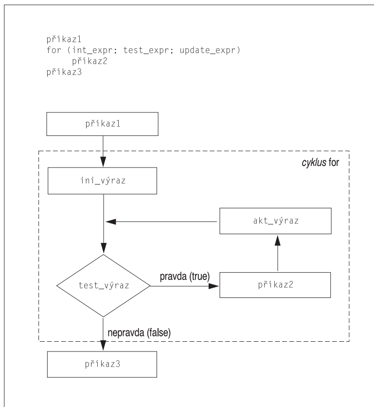
Obrázek 5.1 Cyklus for
