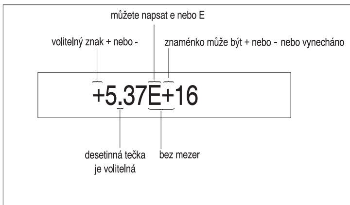
Obrázek 3.3 E notace
