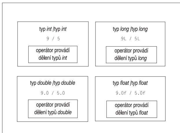
Obrázek 3.4 Různá dělení
