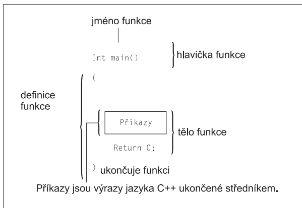
Obrázek 2.1: Funkce main()
