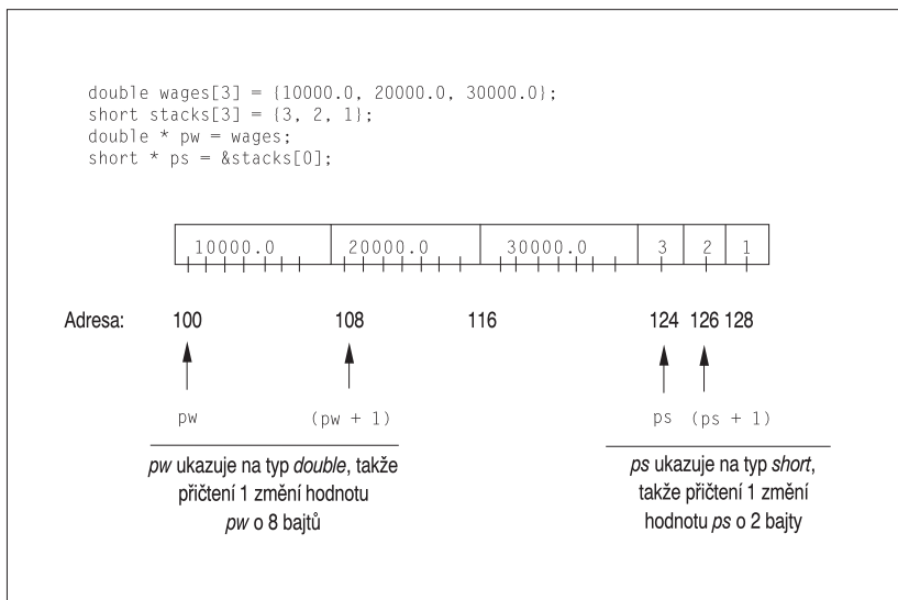
Obrázek 4.10 Sčítání ukazatelů
