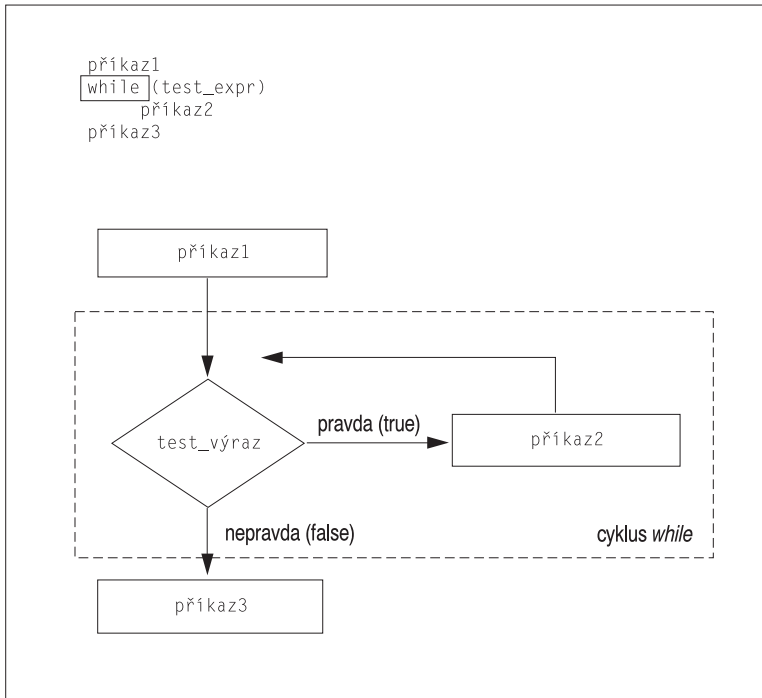
Obrázek 5.3 Cyklus while
