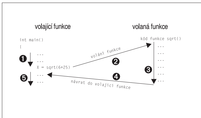
Obrázek 2.6 Volání funkce
