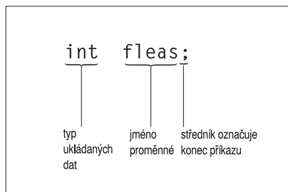
Obrázek 2.4 Deklarace proměnné
